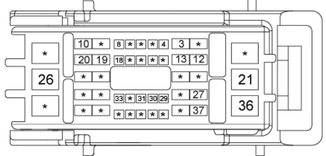
-控制线束
